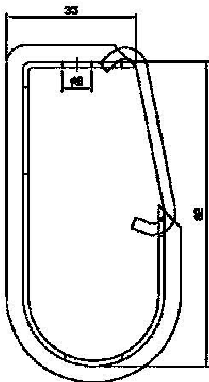
Seitenansicht
